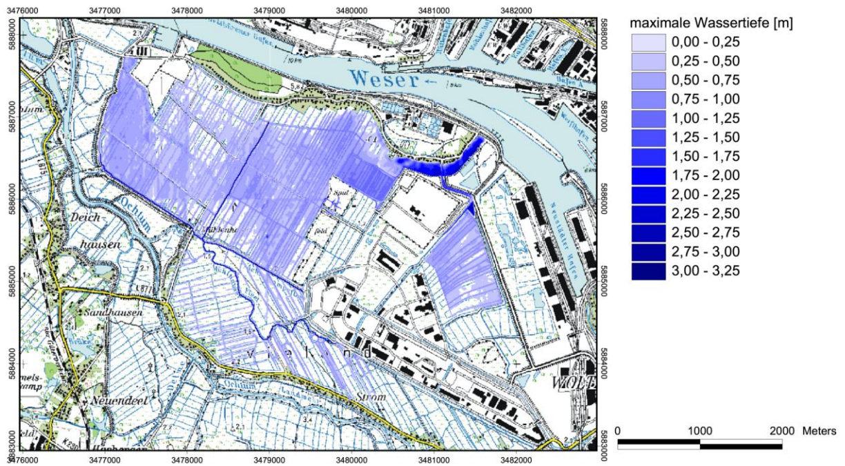
Abb. 5: Maximale Wassertiefen beim Szenario Thw 100 / HQ 100 in der Fokusfläche Seehausen
