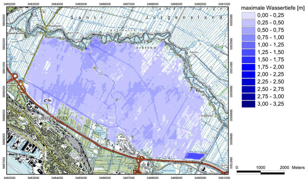
Abb. 7: Maximale Wassertiefen beim Szenario Thw 100 / HQ 100 in der Fokusfläche Blockland
