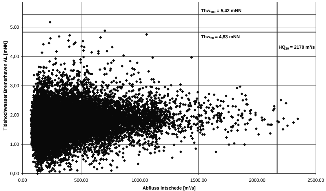
Abb. 2: Gegenüberstellung der Tidehochwasserstände am Pegel Bremerhaven Alter Leuchtturm und der Abflüsse am Pegel Intschede zwischen 1965 und 2004
