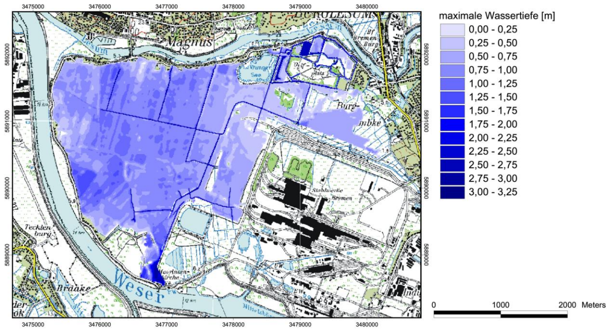
Abb. 3: Maximale Wassertiefen beim Szenario Thw 100 / HQ 100 in der Fokusfläche Werderland
