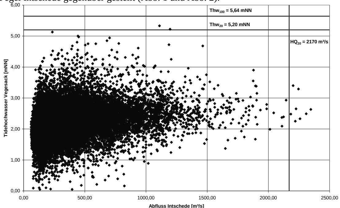
Abb. 1: Gegenüberstellung der Tidehochwasserstände am Pegel Vegesack und der Abflüsse am Pegel Intschede zwischen 1950 und 2003
