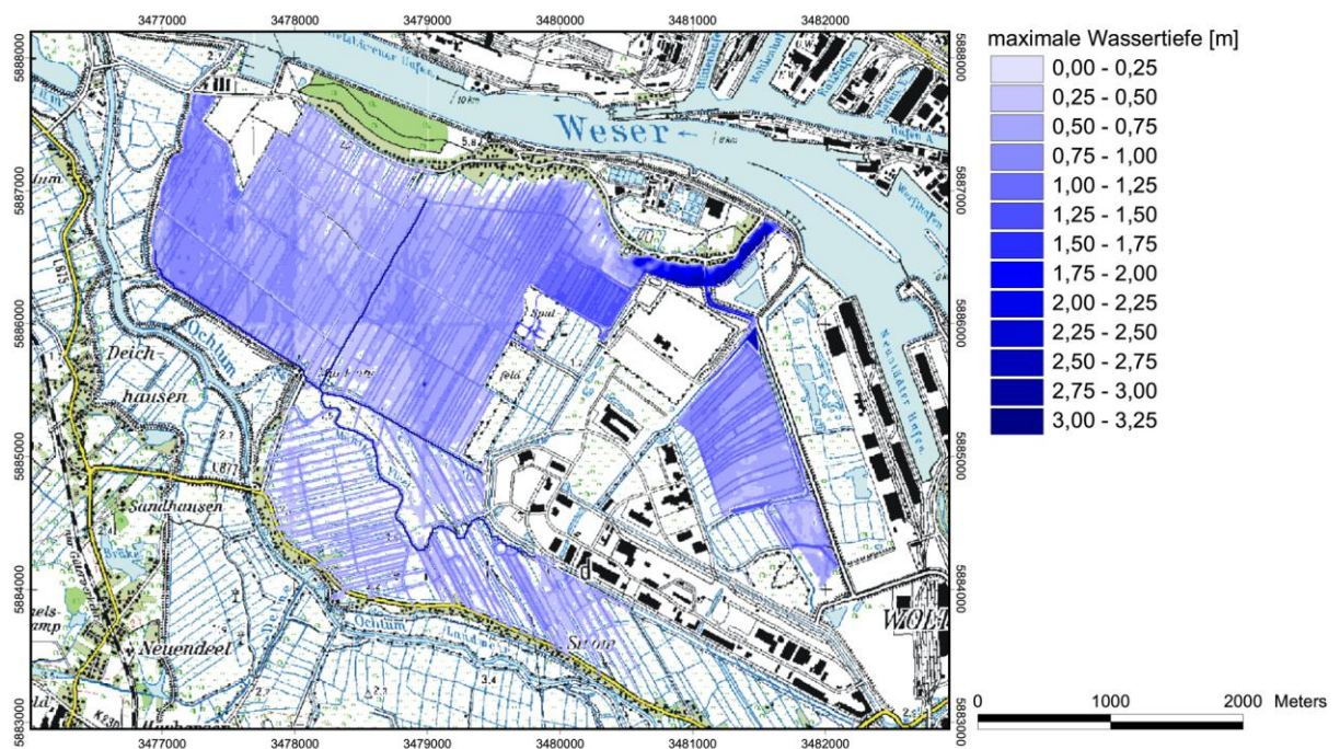
Abb. 6: Maximale Wassertiefen beim Szenario Thw 100 / HQ 100 und einem Anstieg des Meeresspiegels um 55 cm (Klimaszenario) in der Fokusfläche Seehausen
