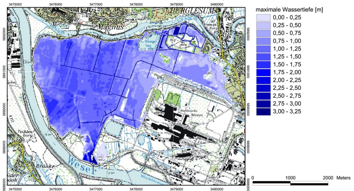
Abb. 4: Maximale Wassertiefen beim Szenario Thw 100 / HQ 100 und einem Anstieg des Meeresspiegels um 55 cm (Klimaszenario) in der Fokusfläche Werderland
