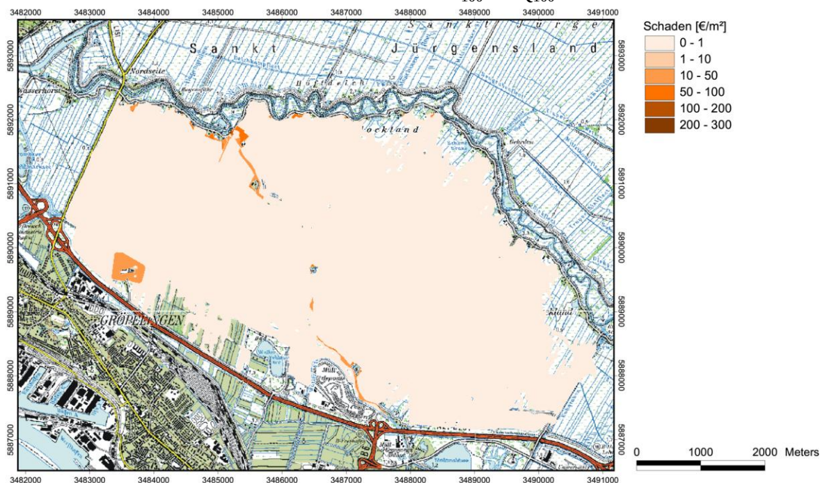
Abb. 8: Schäden beim Szenario Thw 100 / HQ 100 und einem Anstieg des Meeresspiegels um 55 cm (Klimaszenario) in der Fokusfläche Blockland
